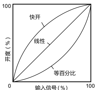
图 4. 输入输出特性
