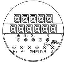
连接端子配置图 (端子螺丝尺寸: M4)
